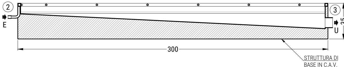
SEZIONE LONGITUDINALE
