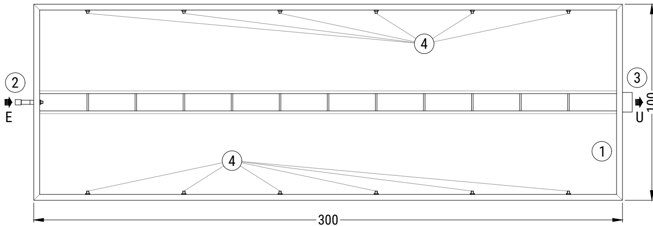
PIANTA
