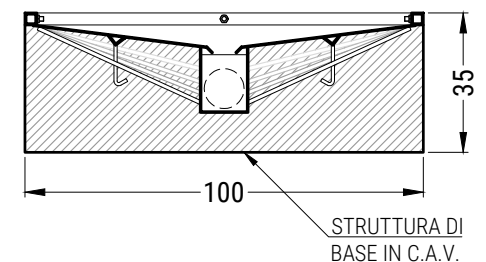
SEZIONE TRASVERSALE
