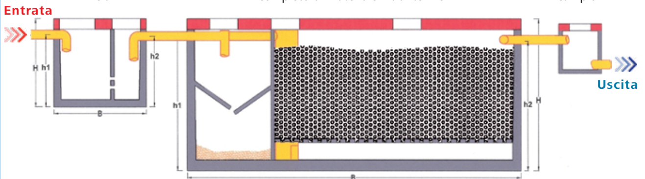
Degrassatore/Separatore in c.a.v.
