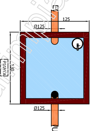
SEPARATORE LIQUIDI PER AUTORIMESSE INTERRATE CON FILTRO A COALESCENZA E SERBATORIO INTERNO IN PVC
