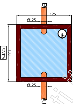
SEPARATORE LIQUIDI PER AUTORIMESSE INTERRATE CON SERBATORIO INTERNO IN PVC
