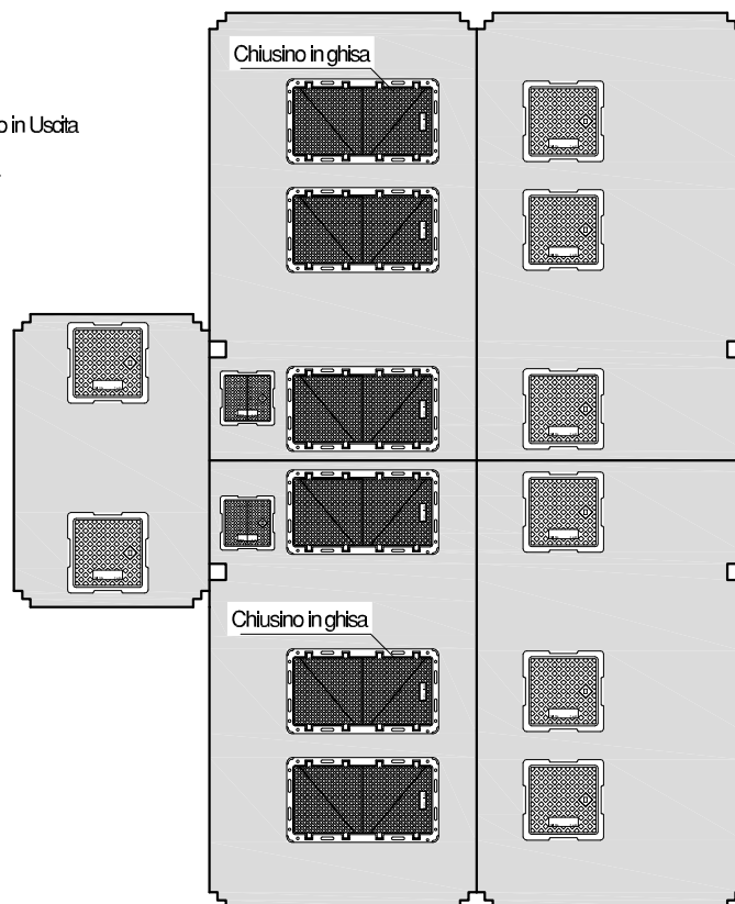
Planimetria - lastre di copertura
